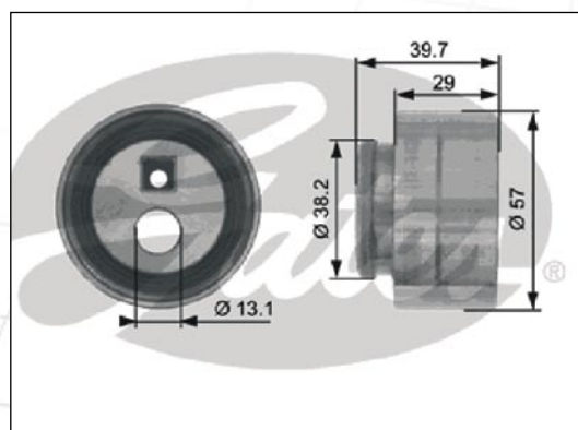
Fig. 1 Tendeur manuel (K025468XS)
