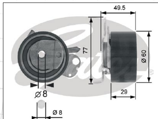
Fig. 2 Tendeur automatique (K035468XS)
